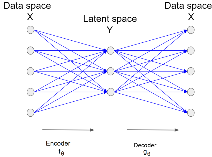
FIGURE 1.4. Autoencoder.
